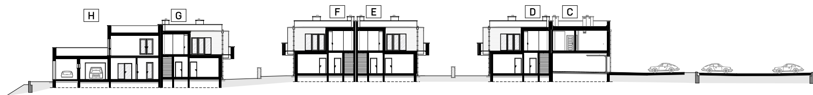
przekrój _ etap 2 skala 1:350
