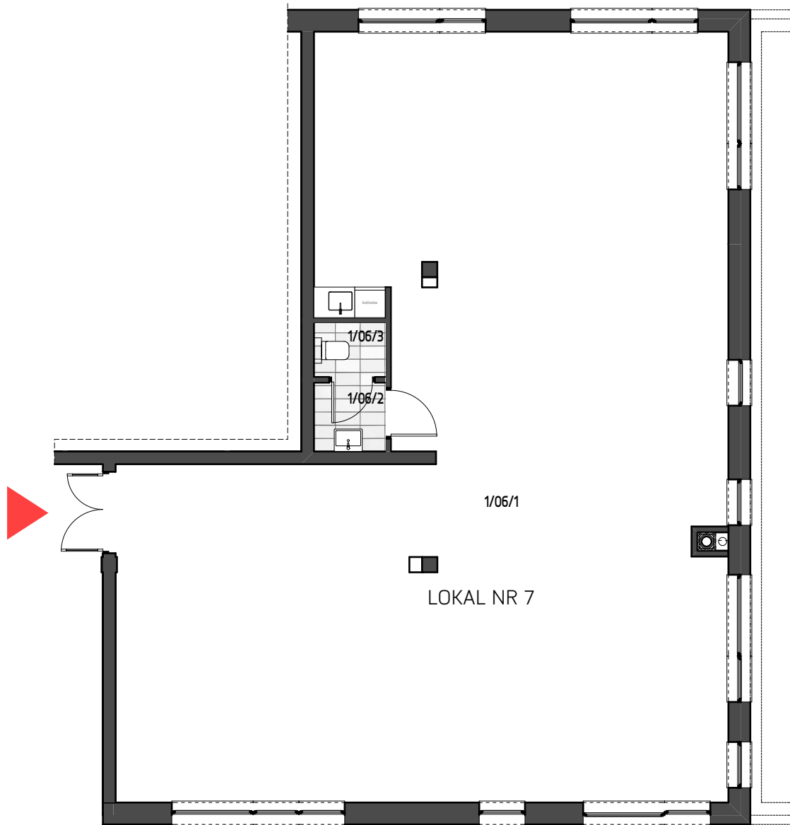
BUDYNEK B Lokal usługowy 7
