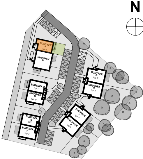
PLAN SYTUACYJNY - SCHEMAT
